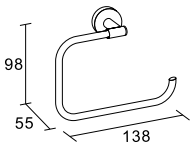
# 740007 Papierrollenhalter Toilet Roll Holder
